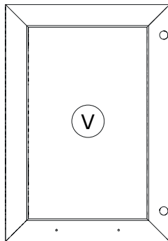
VT0161 733x507x18mm
